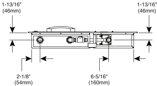
Vista inferior
