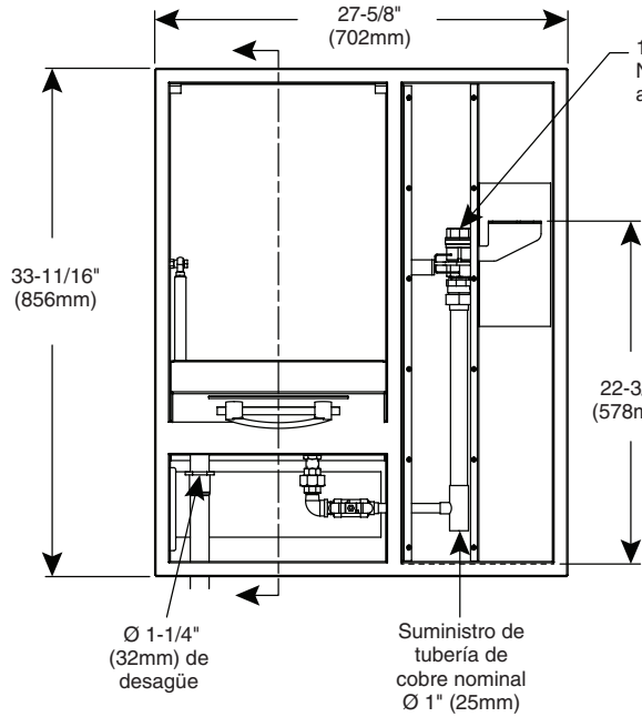
Vista delantera
